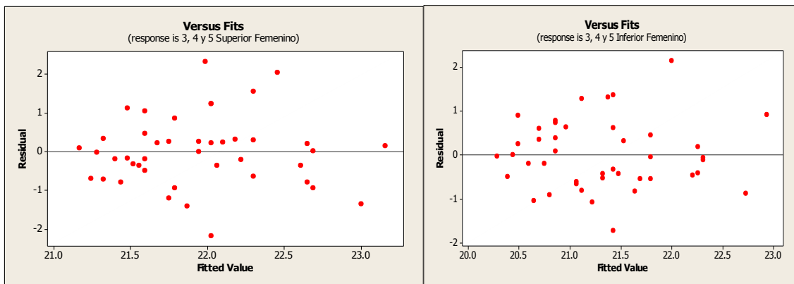
Figura 1. Gráfico de residuos para los ajustes de la ecuación modificada de Tanaka-Johnston para el sexo femenino.
