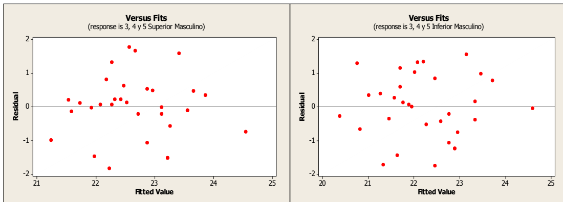
Figura 2. Gráfico de residuos para los ajustes de la ecuación modificada de Tanaka-Johnston para el sexo masculino.
